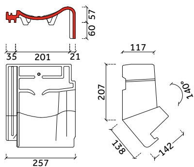
knikgevelpan rechts 140°
