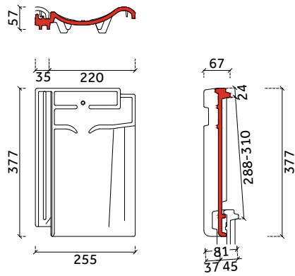
dakpan
