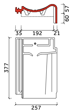
ondergevelpan rechts
