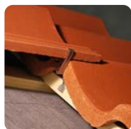
Euro-panhaak Sneldek
