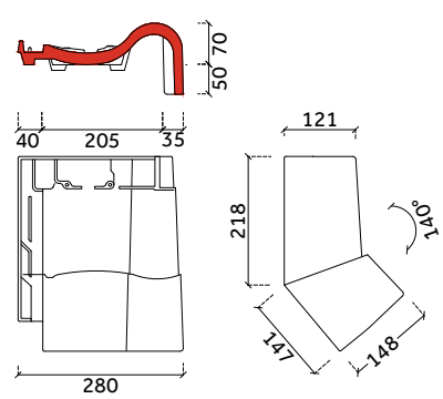
knikgevelpan rechts 140°
