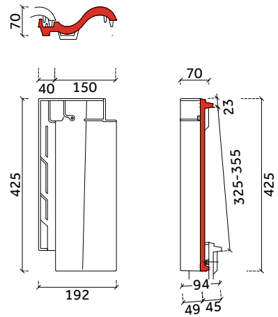
2/3 pan
