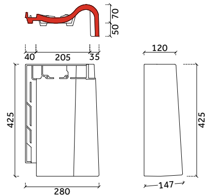
gevelpan rechts
