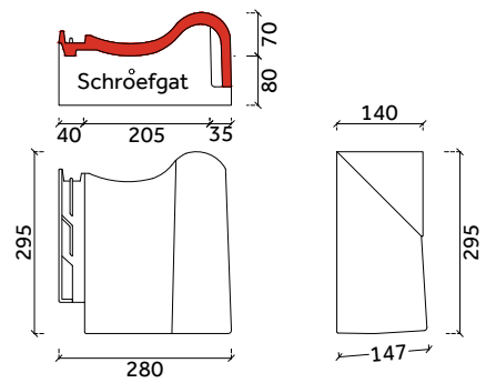
chaperongevelpan rechts 90°
